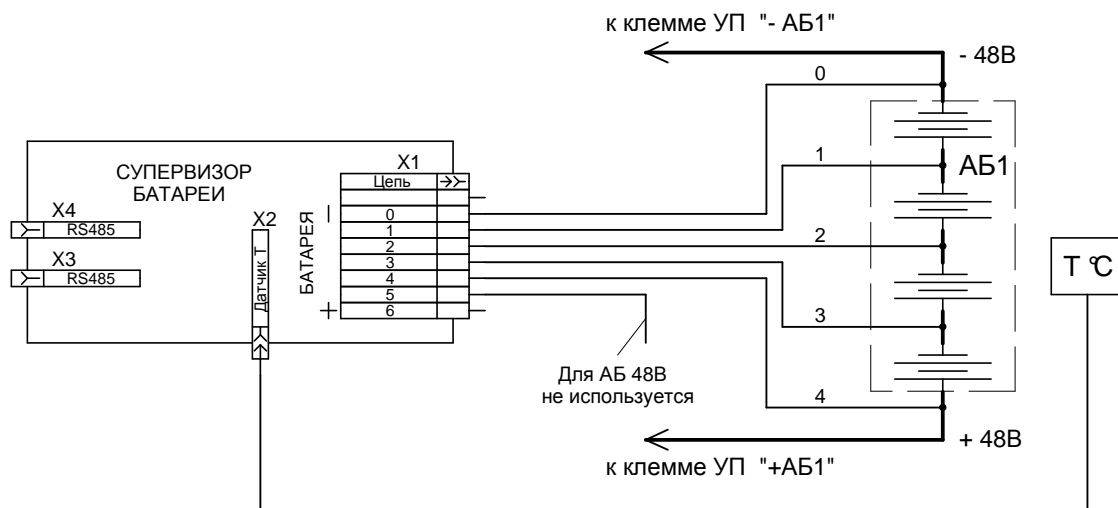
Рисунок 2.2 – Схематичное изображение подключения модуля САБ
