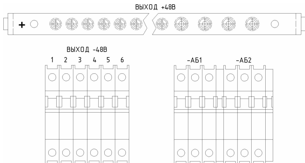
Рисунок 2.1 – Подключение нагрузки и аккумуляторных батарей
